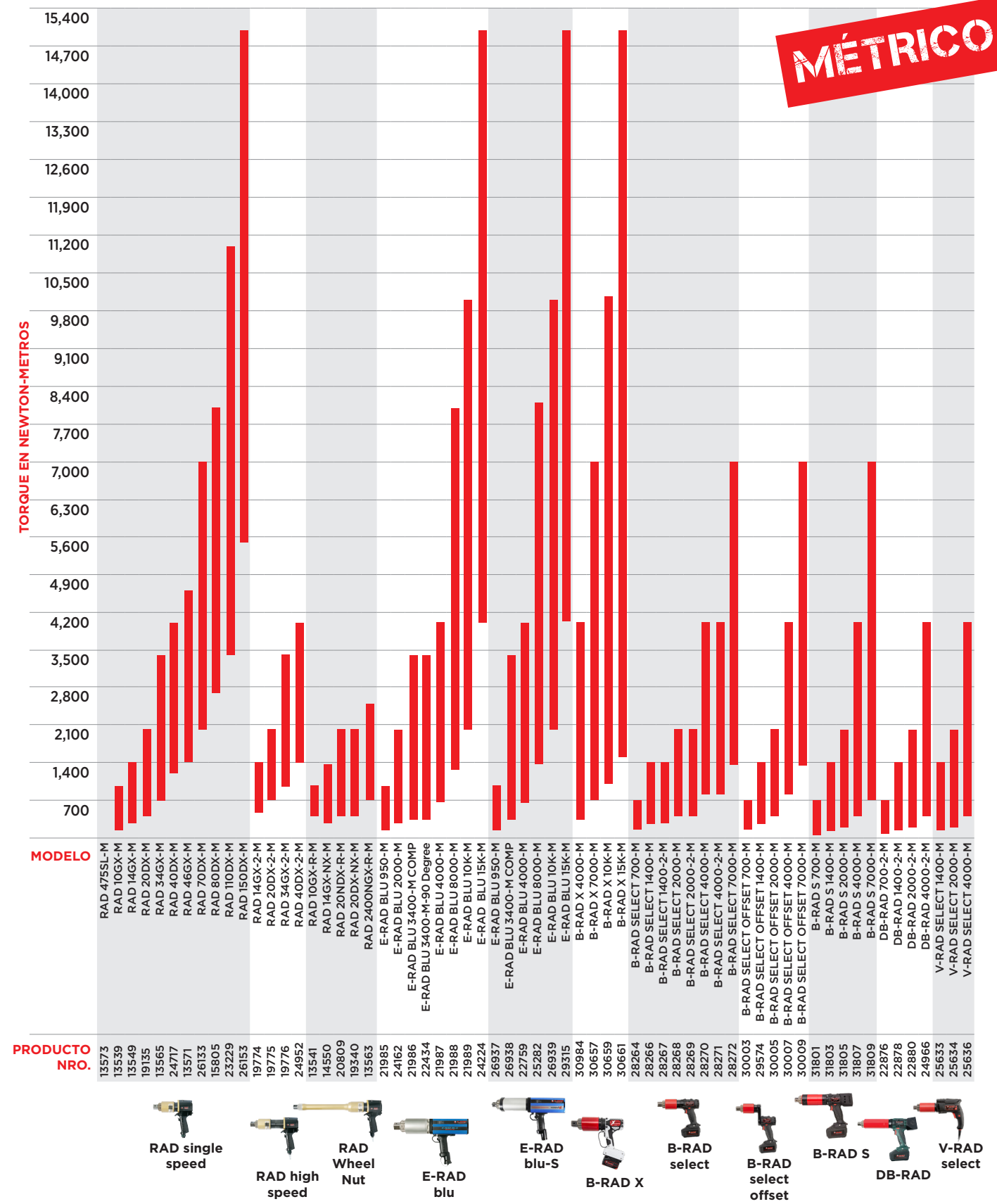
LLAVE DE TORQUE
