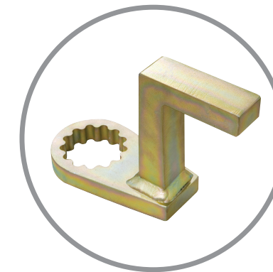
BRAZO DE REACCIÓN PARA DADO PROFUNDO
